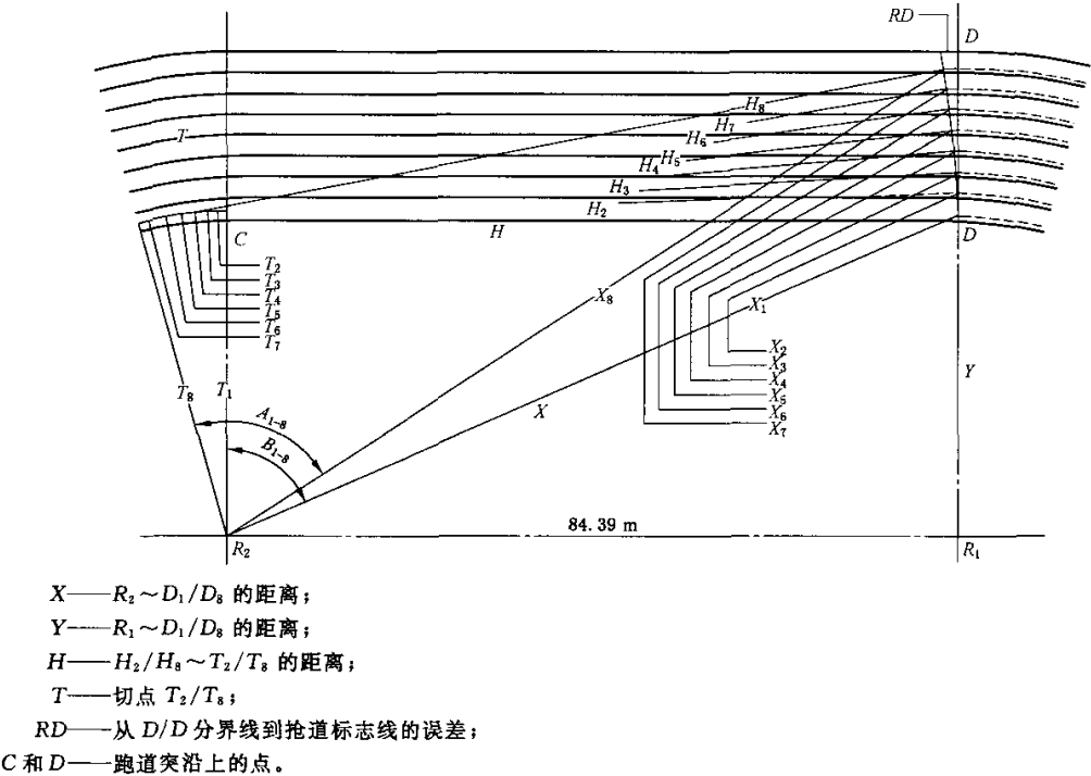
图 A.1 400 m 标准跑道 800 m 跑抢道标志线
