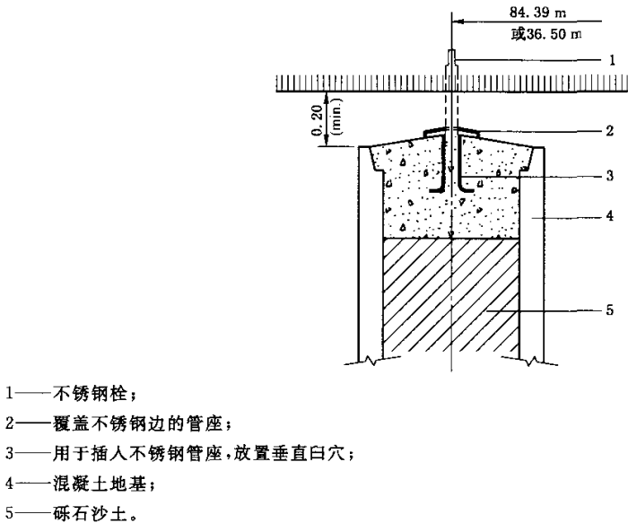
图 B.2 基准桩构造
