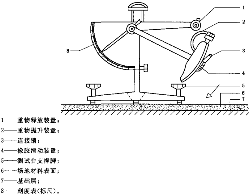
图 F.1 便携式阻力测试仪
