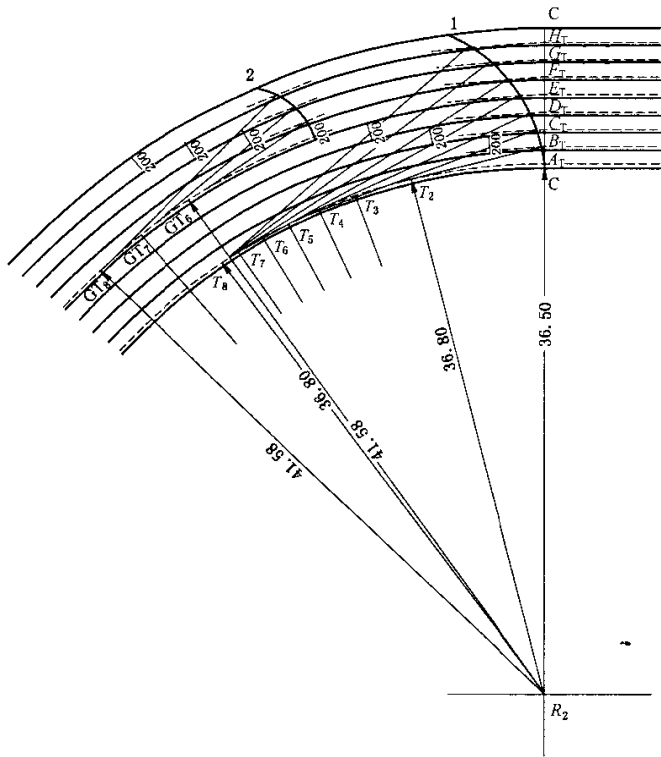
1——1 000 m、3 000 m 和 5 000 m 的起点线； 2——1 000 m、3 000 m 和 5 000 m 的分组起跑线。 注：R 2 C——36.50 m；R 2 A T ——36.80 m；R 2 B T ——36.80 m + 1.12 m；R 2 G T …H T ——37.92 m + 每道 1.22 m； T 2 T 8 ——切线点；G T G T ——分组起跑线的切线点。
