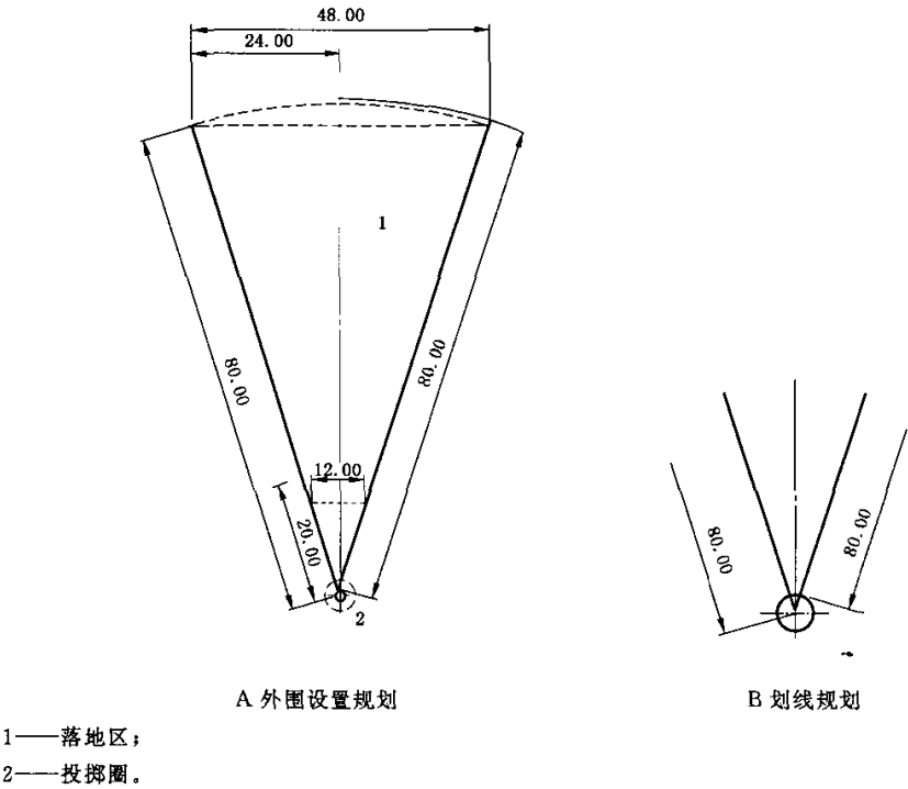
图 A.12 掷铁饼设施
