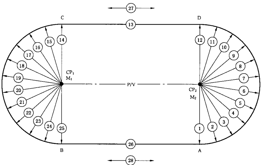
图 5 400 m 跑道精确测量点位示意图
