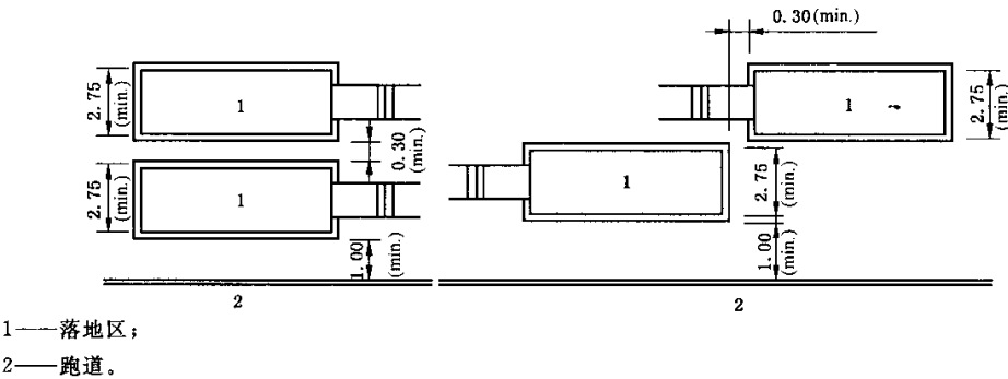
b) 两个平行的跳远与三级跳远设施间的最小距离
