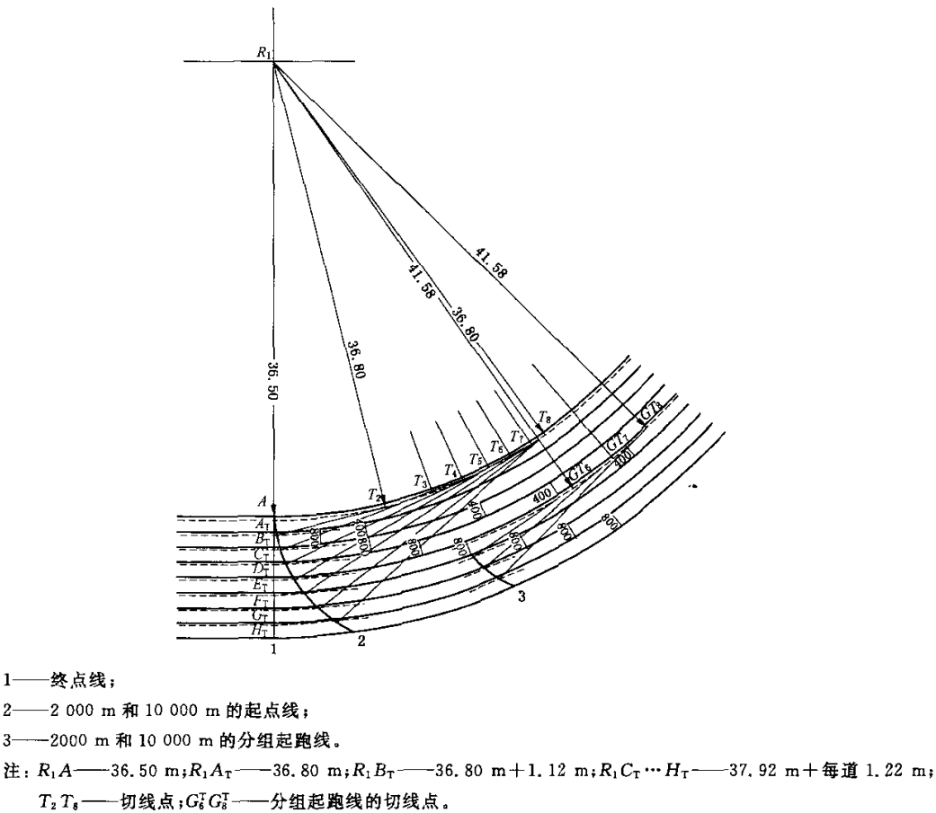
图 A. 2 400 m 标准跑道第一弯道上的 2 000 m 和 10 000 m 起点线和分组起跑线
