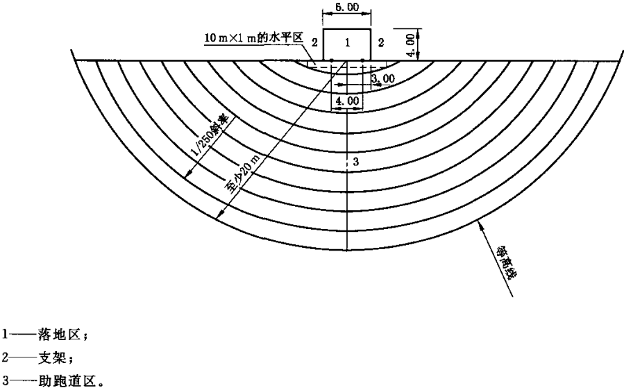
图 A.6 跳高设施
