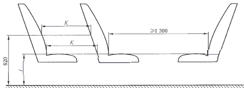
图 12 座椅间距
