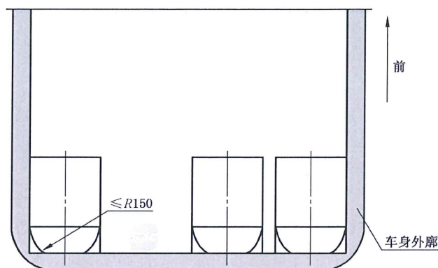
图 16 最后一排外侧座位空间的允许侵入
