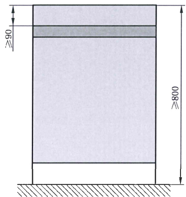
图 17 驾驶区后面乘客座位挡板示意图
