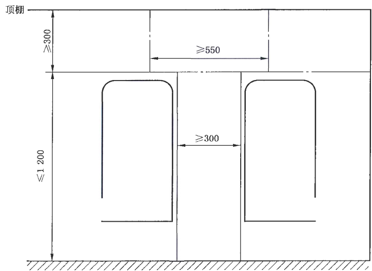
图 6 至车门的无障碍通路(横轴方向)
