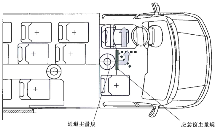
图 2 驾驶区对主乘客区乘员的通过性
