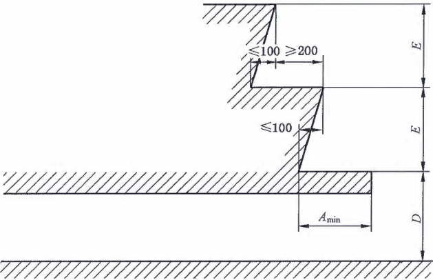
图 11 乘客用踏步
