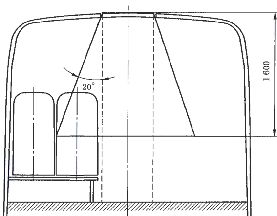
图8 安全顶窗校核
