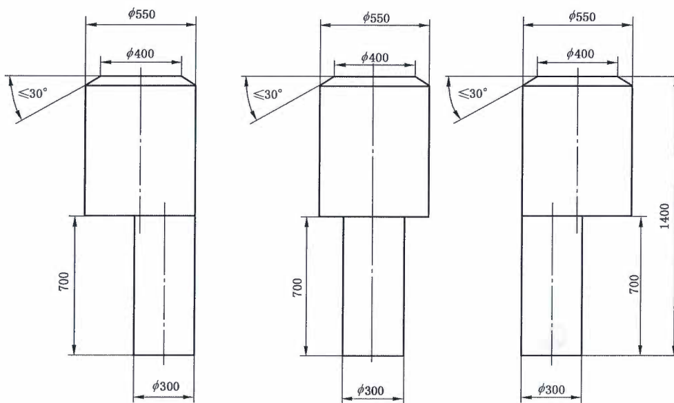
图 7 应急门引道量规
