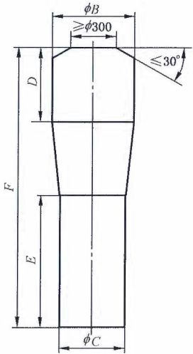
图 9 通道主量规
