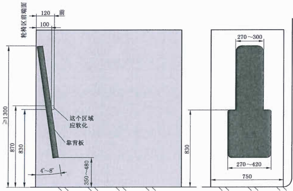
图 A.5 靠背尺寸示意图
