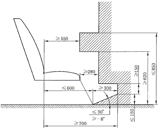
图 13 隔离物后的乘客座位前方自由空间
